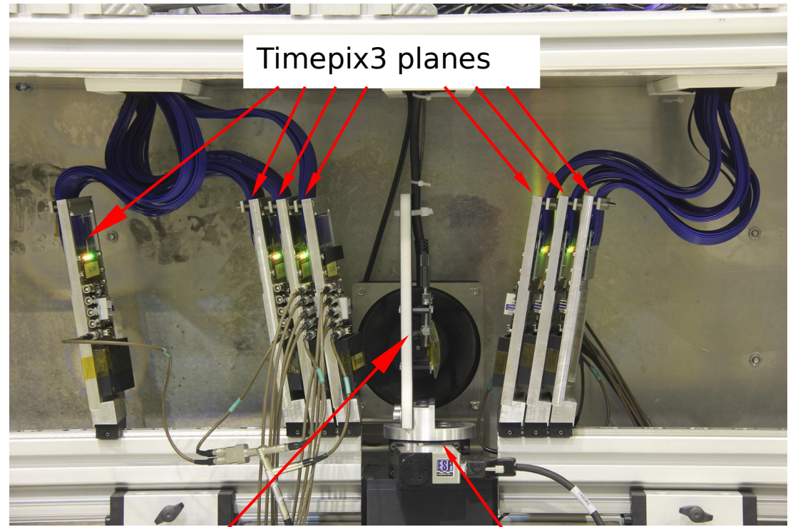
device-under-test (DUT)
