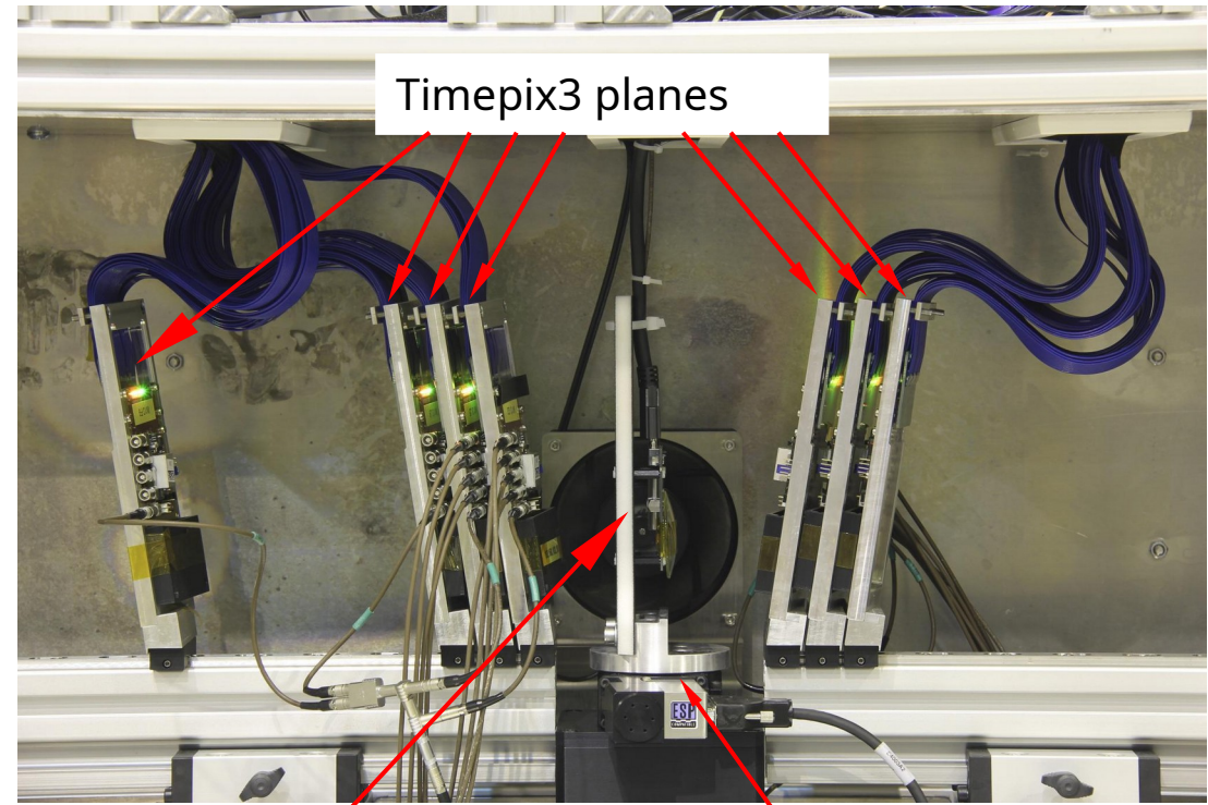
device-under-test (DUT)
