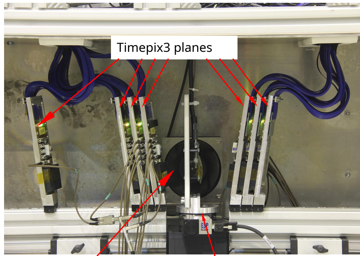
device-under-test (DUT)
